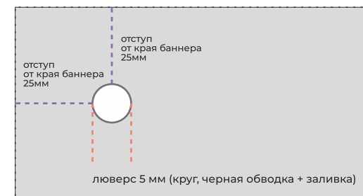
схема расстановки люверсов (для примера взят левый верхний угол)
